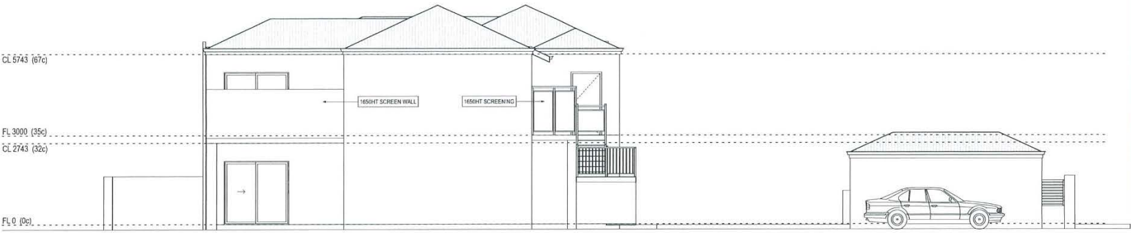
ELEVATION 3 SCALE: 1:100
